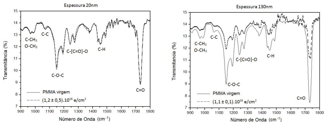
Figura 09 – Espectros de PMMA de diferentes espessuras, antes e depois de serem irradiados com elétrons.
